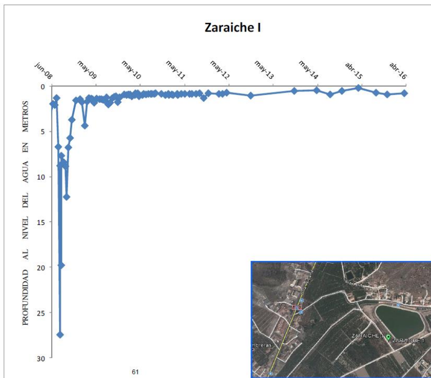
Figura 11. Evolución del nivel de agua en el pozo de sequía de Zaraiche I
