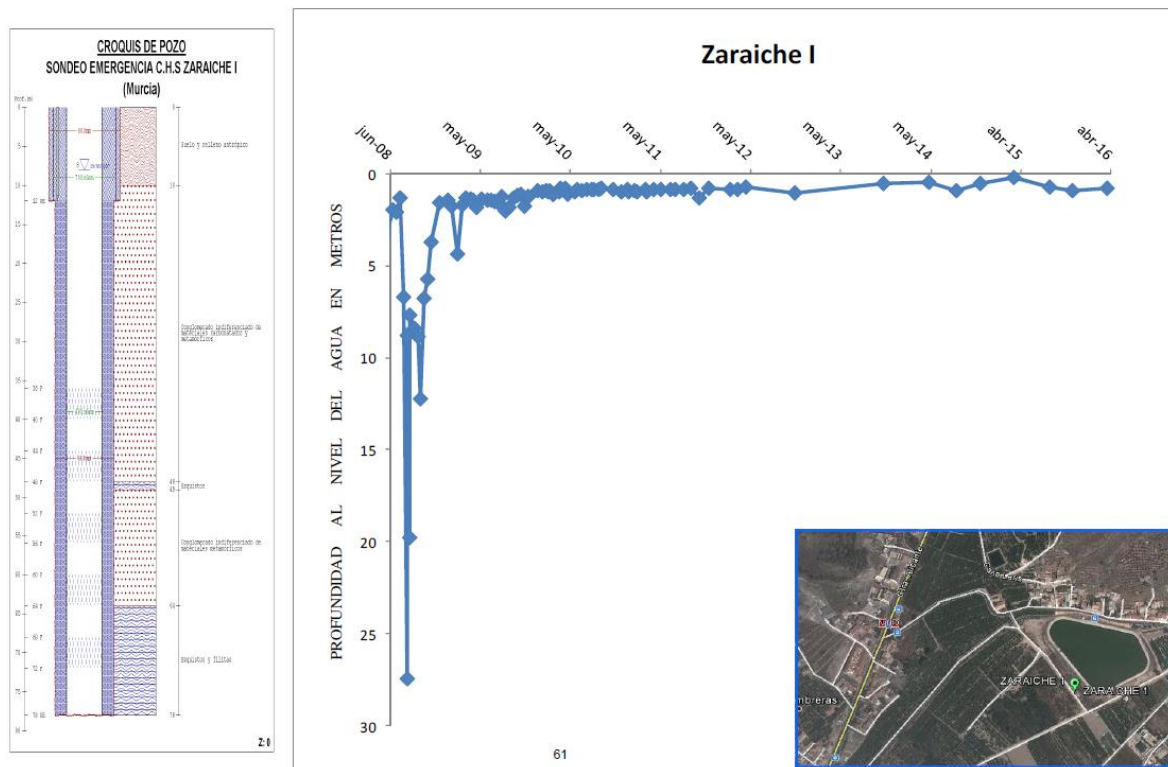
Figura 3. Evolución del nivel de agua en el pozo de sequía de Zaraiche I
