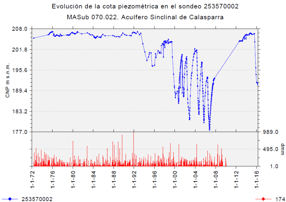
Figura 16. Evolución del nivel piezométrico en el sondeo 253570002, punto de control de la masa Acuífero Sinclinal de Calasparra
