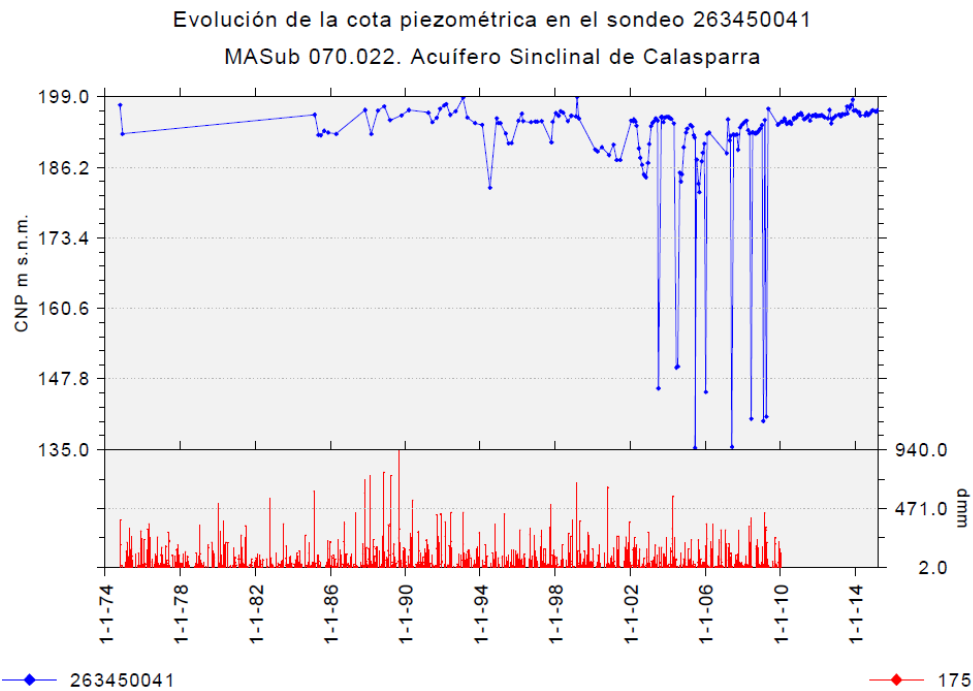
Figura 18. Evolución del nivel piezométrico en el sondeo 263450041, punto de control de la masa de agua Acuífero Sinclinal de Calasparra
