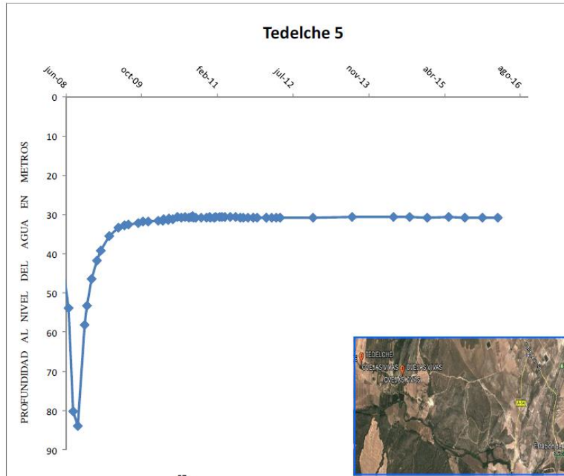
Figura 10. Evolución del nivel de agua en el pozo de sequía de Tedelche 5
