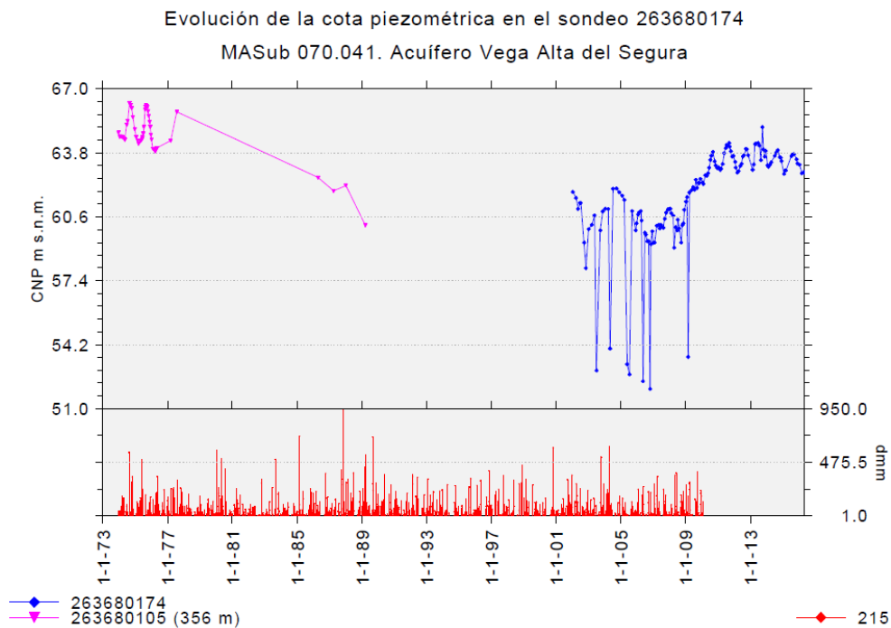
Figura 20. Evolución del nivel piezométrico en el sondeo 263680174, punto de control de la masa de agua Acuífero Vega Alta del Segura
