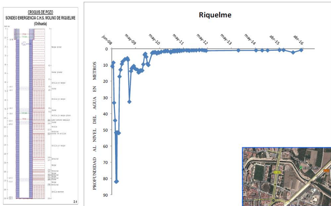
Figura 14. Evolución del nivel de agua en el pozo de sequía de Riquelme
