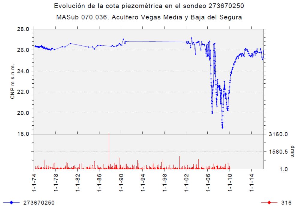
Figura 23. Evolución del nivel piezométrico en el sondeo 273670250, punto de control de la masa de agua Acuífero Vegas Media y Baja del Segura
