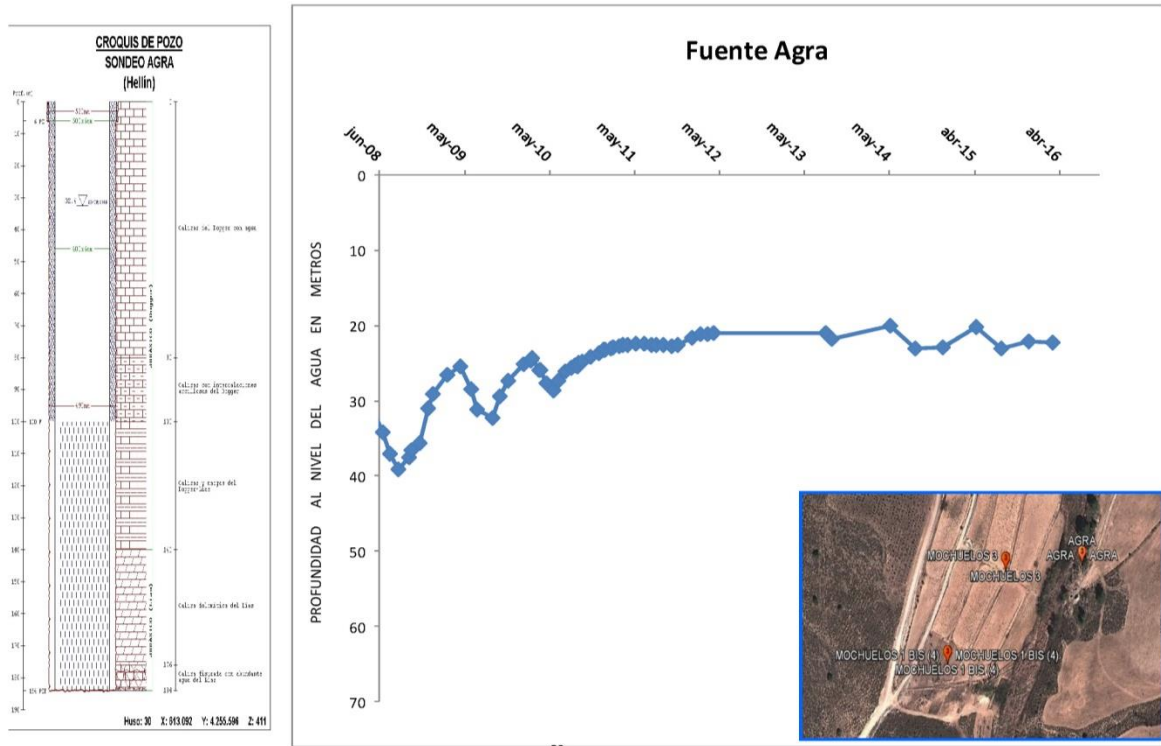
Figura 2. Evolución del nivel de agua en el pozo de sequía de Fuente Agra
