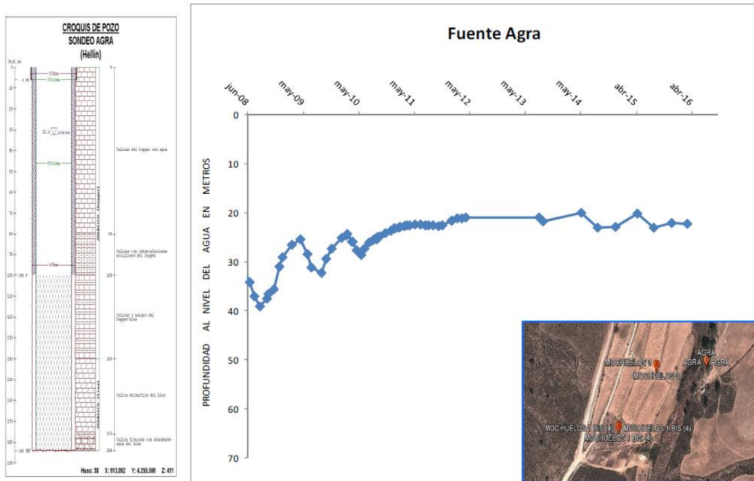
Figura 9. Evolución del nivel de agua en el pozo de sequía de Fuente Agra
