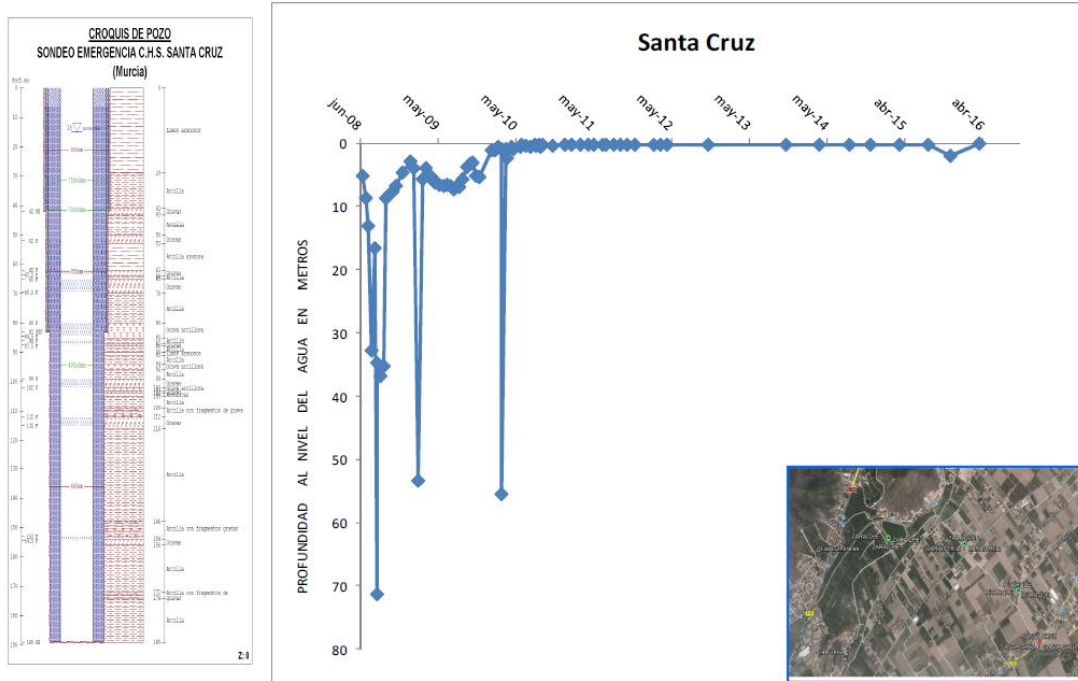
Figura 12. Evolución del nivel de agua en el pozo de sequía de Santa Cruz
