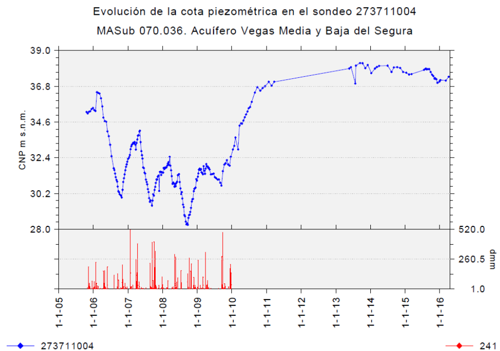
Figura 24. Evolución del nivel piezométrico en el sondeo 273711004, punto de control de la masa de agua Acuífero Vegas Media y Baja del Segura
