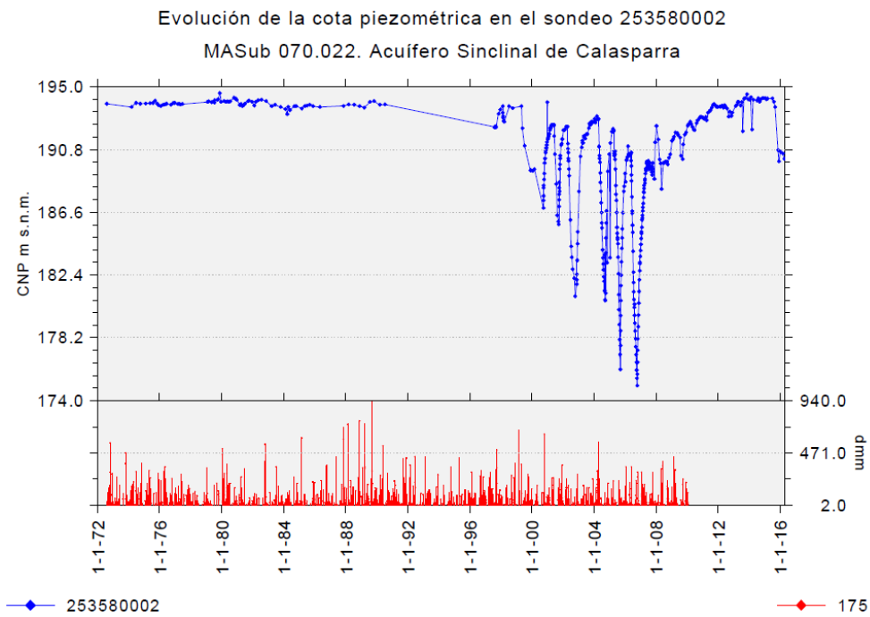
Figura 17. Evolución del nivel piezométrico en el sondeo 253580002, punto de control de la masa de agua Acuífero Sinclinal de Calasparra
