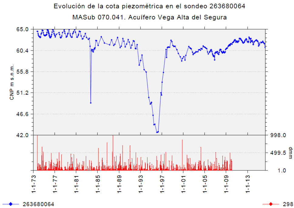
Figura 19. Evolución del nivel piezométrico en el sondeo 263680064, punto de control de la masa de agua Acuífero Vega Alta del Segura
