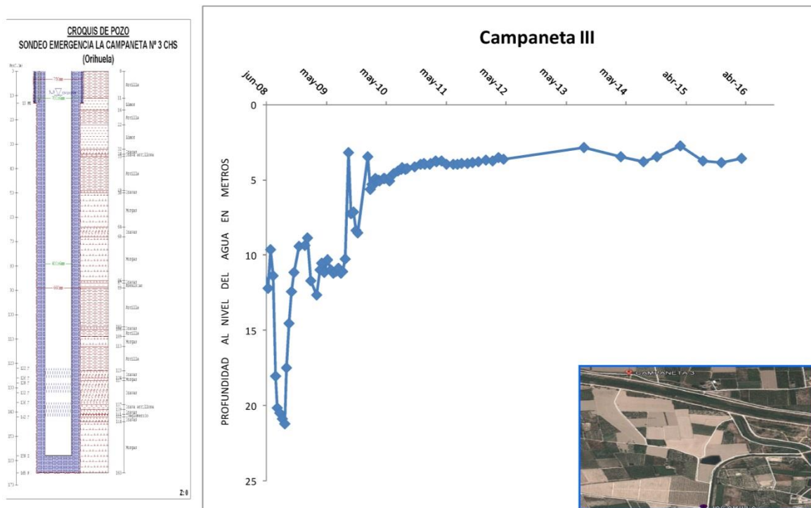
Figura 4. Evolución del nivel de agua en el pozo de sequía de Campaneta III
