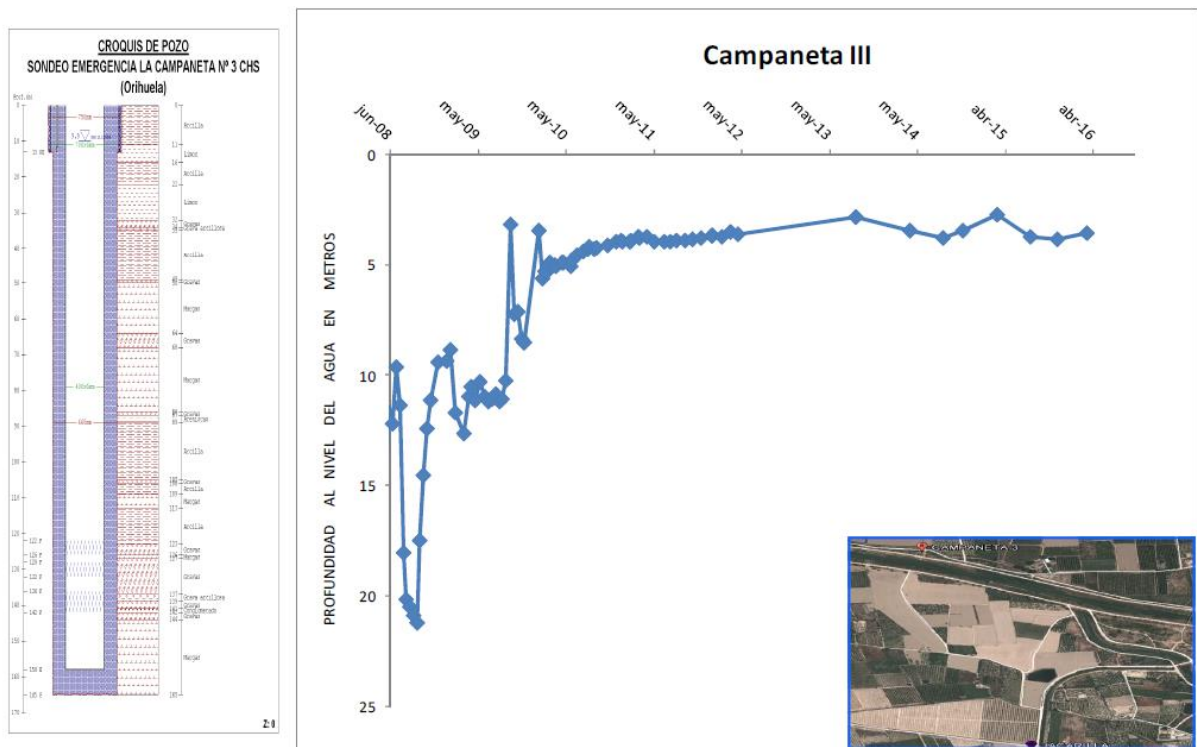
Figura 13. Evolución del nivel de agua en el pozo de sequía de Campaneta III
