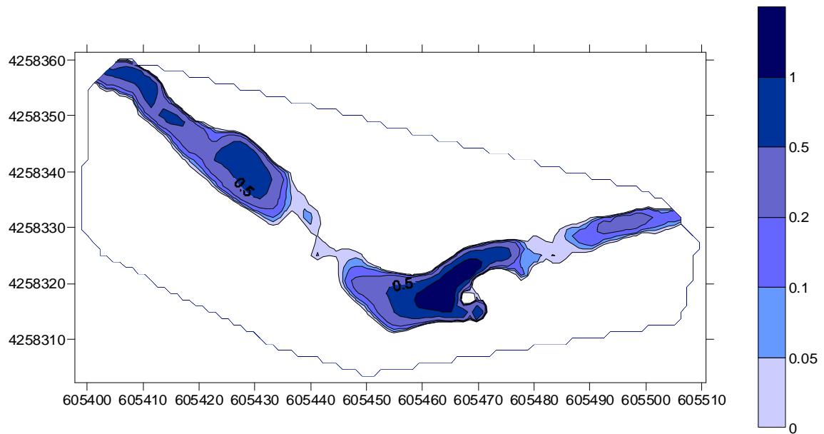
Figura 20. Calados para el caudal de los modelados donde se observa pérdida de continuidad en tramo de la masa de agua ES0701010304 ( 0,05 \text{ m}^3/\text{sg} )
