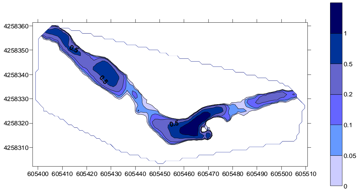
Figura 19. Calados para el caudal de los modelados anterior al que presenta la pérdida de continuidad en tramo de la masa de agua ES0701010304 ( 0,11 \text{ m}^3/\text{sg} ).
