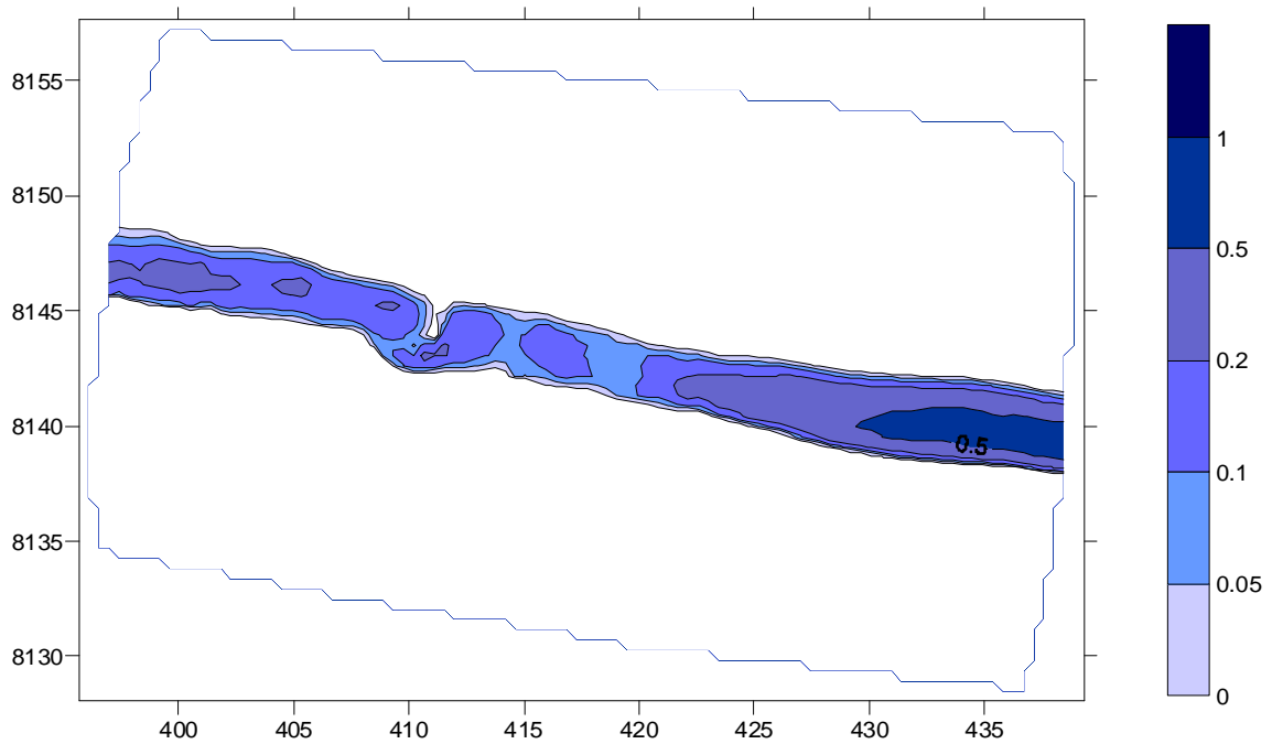
Figura 26. Calados para el caudal 0,15 m 3 /sg en tramo de la masa de agua ES0701011801 y ES0701011802
