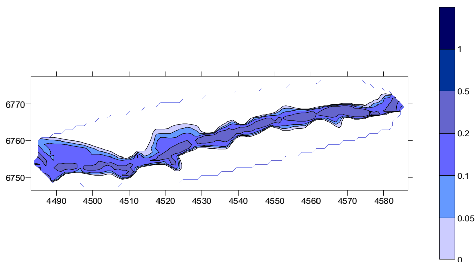
Figura 24. Calados para el caudal 0,5 m 3 /sg en tramo de la masa de agua ES0701011103
