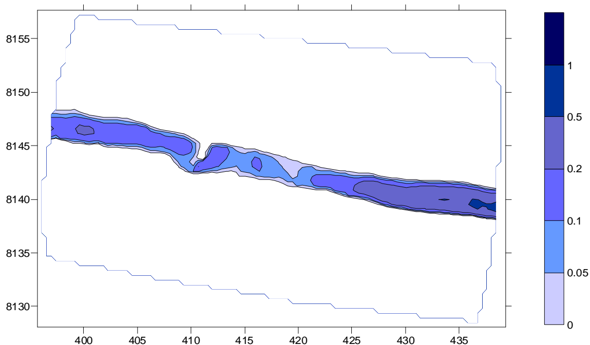
Figura 27. Calados para el caudal de los modelados anterior al que presenta pérdida de continuidad en tramo de la masa de agua ES0701011801 y ES0701011802 ( 0,1 \text{ m}^3/\text{sg} )
