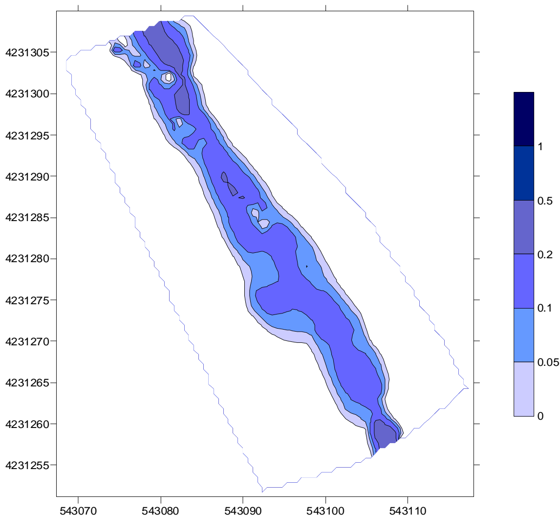
Figura 4. Calados para el caudal 0,4 m 3 /sg en tramo de la masa de agua ES0701010103.
