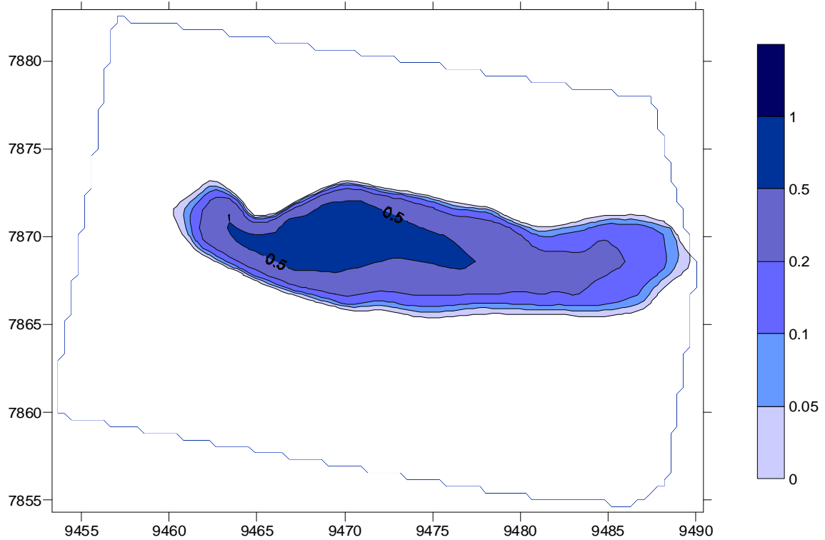
Figura 23. Calados para el caudal de los modelados donde se observa pérdida de continuidad en tramo de la masa de agua ES0701010401 ( 0,01 \text{ m}^3/\text{sg} )
