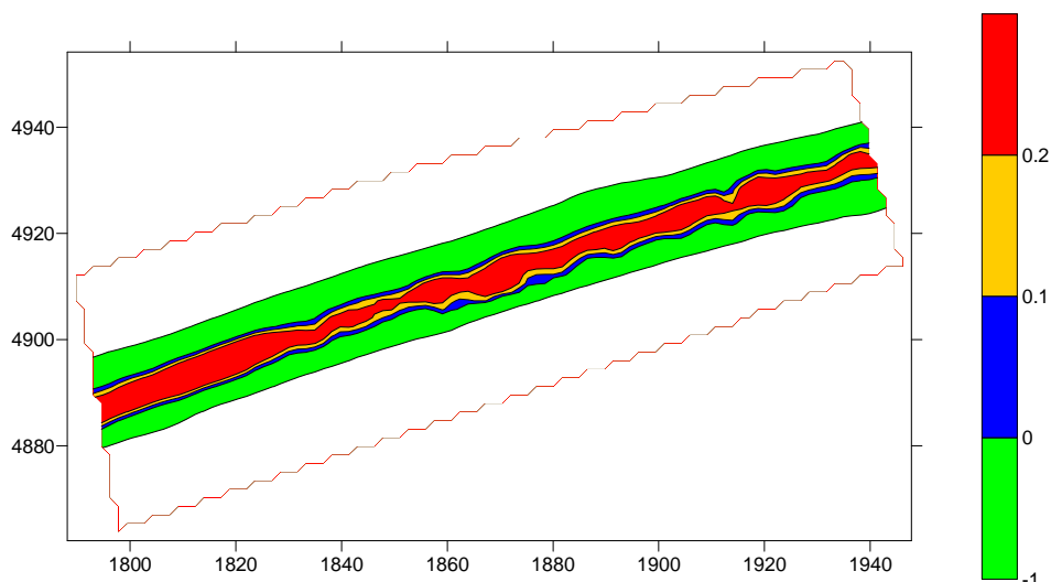
Figura 38. Calados para el caudal 0,3 m 3 /sg en tramo de la masa de agua ES0702080115
