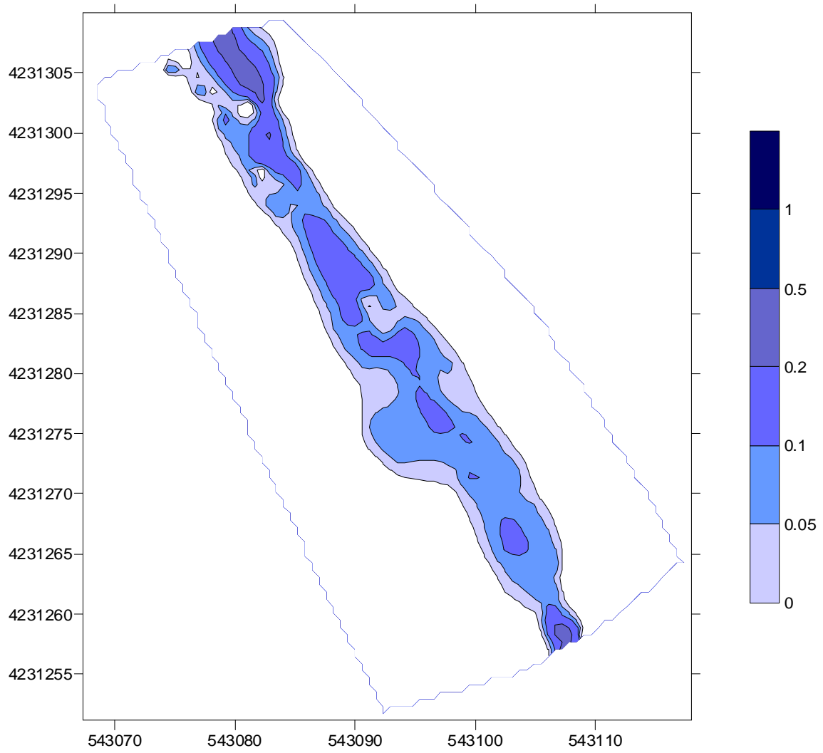
Figura 5. Calados para el caudal menor de los modelados, 0,2 \text{ m}^3/\text{sg} , donde no se observa pérdida de continuidad en tramo de la masa de agua ES0701010103.
