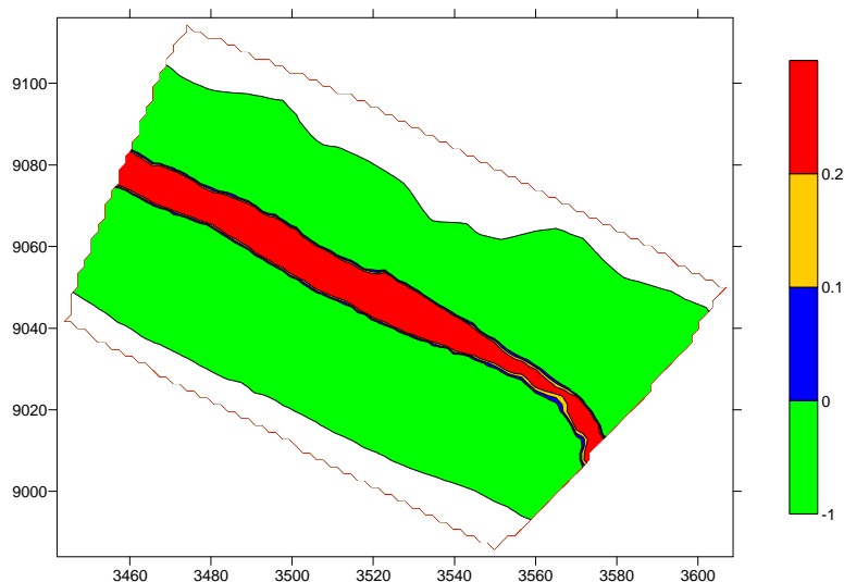
Figura 40. Calados para el caudal 0,3 m 3 /sg en tramo de la masa de agua ES0702080116
