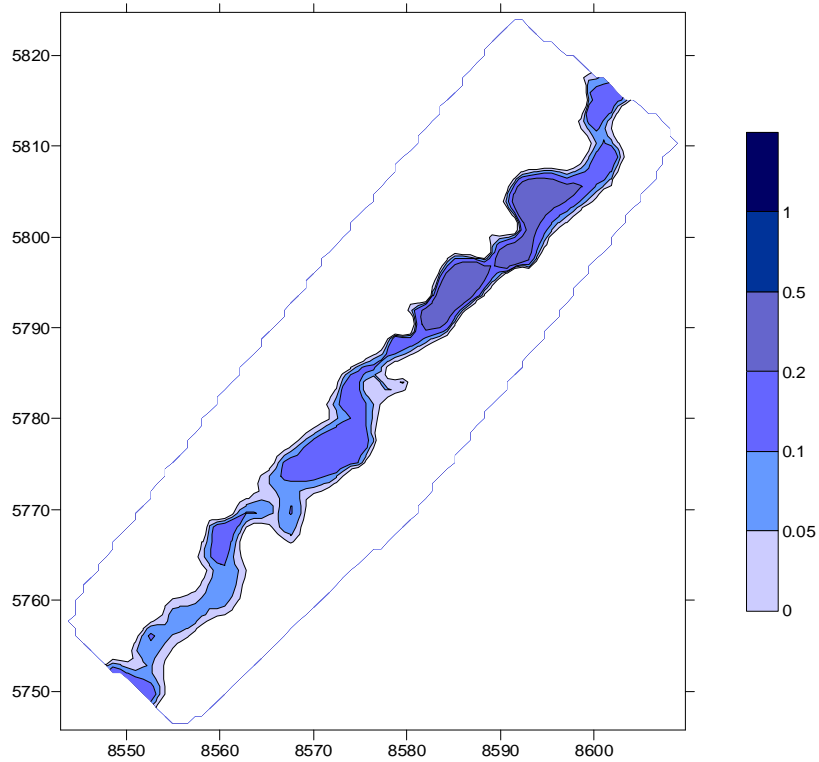
Figura 2. Calados para el caudal de los modelados anterior al que presenta la pérdida de continuidad en tramo de la masa de agua ES0701010101 ( 0,11 \text{ m}^3/\text{sg} )
