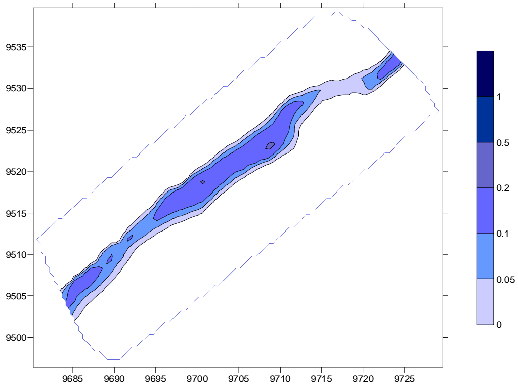
Figura 34. Calados para el caudal de los modelados anterior al de los modelados que presenta pérdida de continuidad en tramo de la masa de agua ES0701012002 ( 0,04 \text{ m}^3/\text{sg} )
