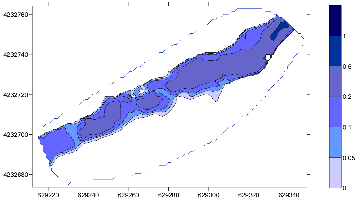
Figura 9. Calados para el caudal 1,2 m 3 /sg en tramo de la masa de agua ES0701010111.
