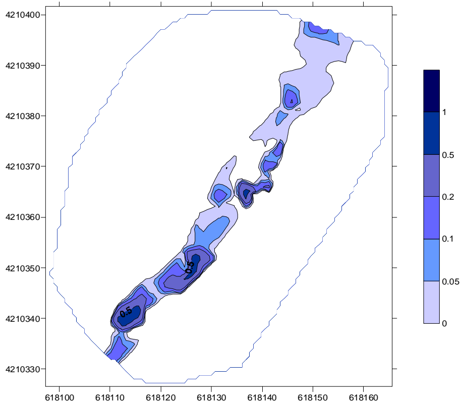
Figura 37. Calados para el caudal de los modelados anterior al que presenta pérdida de continuidad en el tramo de la masa de agua ES0701012304 ( 0,2 \text{ m}^3/\text{sg} )
