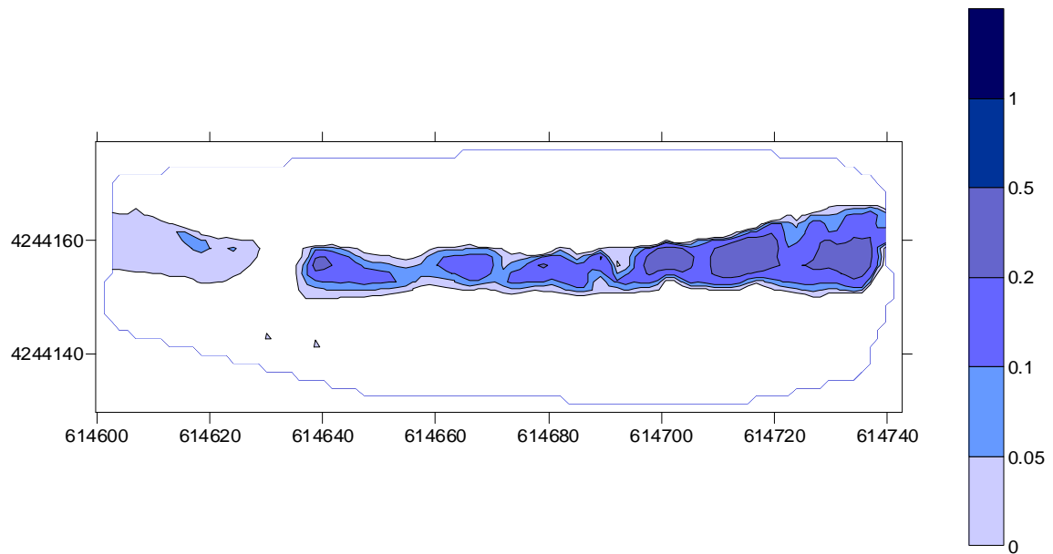
Figura 8. Calados para el caudal de los modelados que produce pérdida de continuidad en tramo de la masa de agua ES0701010109 ( 0,1 \text{ m}^3/\text{sg} ).
