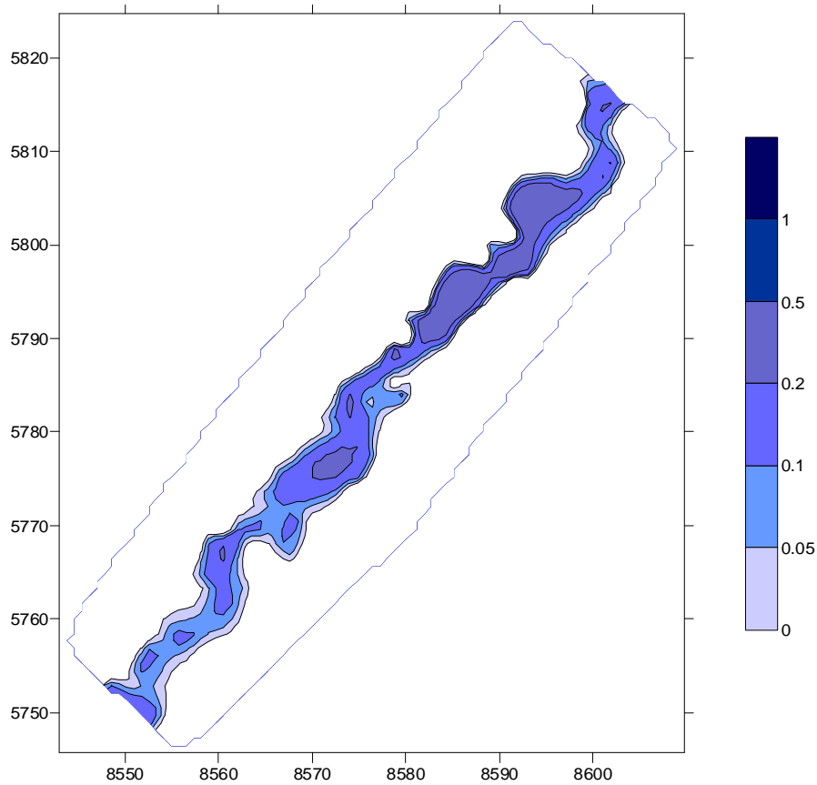
Figura 1. Calados para el caudal 0,15 m 3 /sg en tramo de la masa de agua ES0701010101
