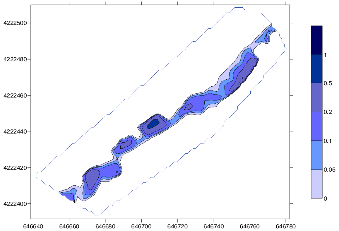
Figura 12. Calados para el caudal menor modelado, 0,1 \text{ m}^3/\text{sg} , en el tramo representativo de las masa de agua ES0701010113
