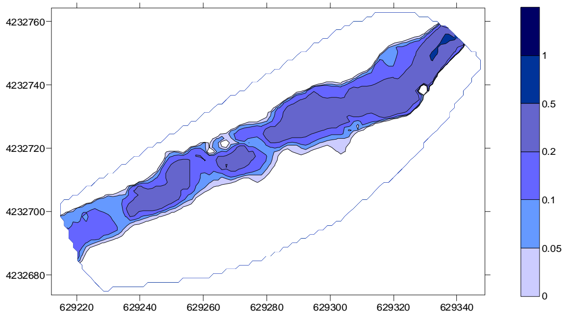
Figura 10. Calados para el caudal menor modelado 1 \text{ m}^3/\text{sg} en el tramo de la masa de agua ES0701010111, donde no se aprecia pérdida de continuidad.
