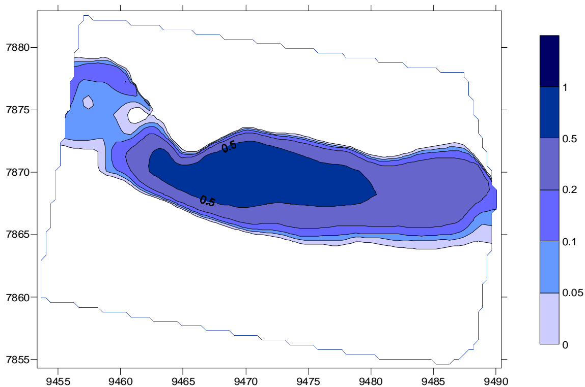
Figura 21. Calados para el caudal 0,2 m 3 /sg en tramo de la masa de agua ES0701010401
