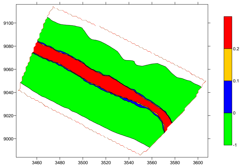
Figura 41. Calados para el caudal 1 \text{ m}^3/\text{sg} en tramo de la masa de agua ES0702080116
