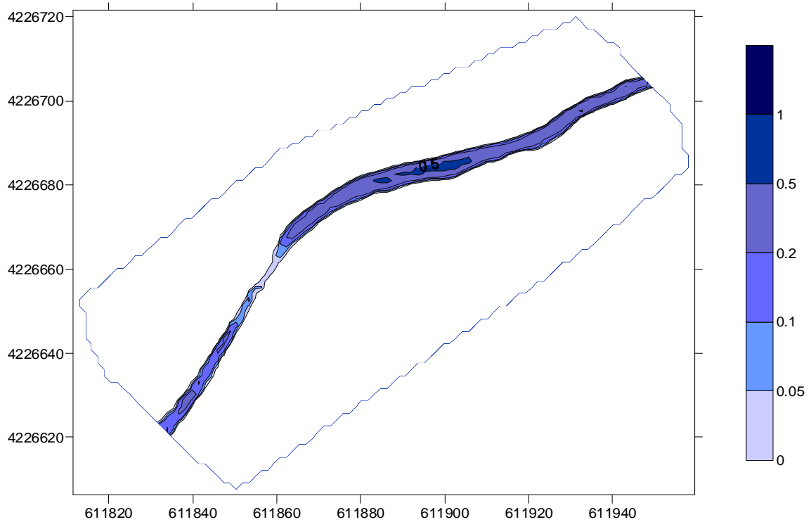
Figura 31. Calados para el caudal 0,1 m 3 /sg, que coincide con el caudal anterior al de los modelados en los que se observa pérdida de continuidad, en tramo de la masa de agua ES0701011903
