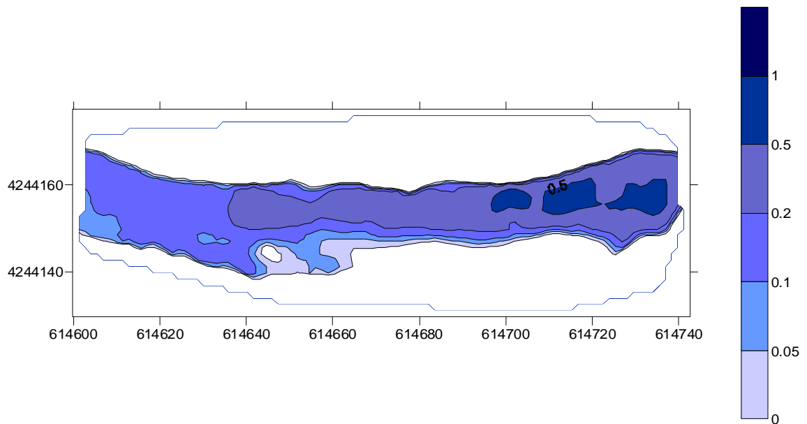
Figura 6. Calados para el caudal 1,4 m 3 /sg en tramo de la masa de agua ES0701010109.
