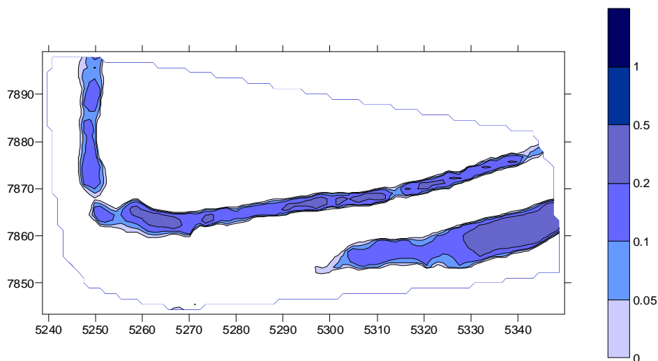
Figura 30. Calados para el caudal de los modelados donde se observa pérdida de continuidad en tramo de la masa de agua ES0701011901 (0,1 m 3 /sg)
