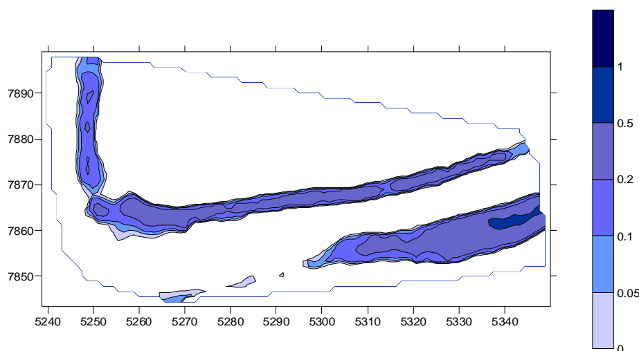
Figura 29. Calados para el caudal 0,15 m 3 /sg (coincide con el caudal anterior al de los modelado en los que se observa pérdida de continuidad) en tramo de la masa de agua ES0701011901.
