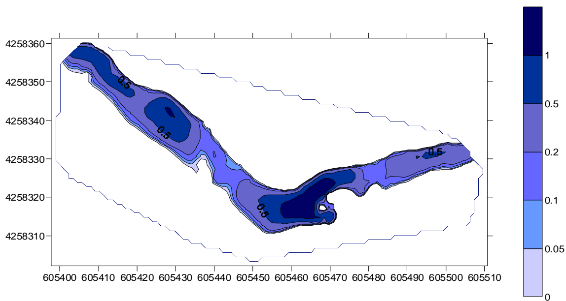
Figura 18. Calados para el caudal 0,5 m 3 /sg en tramo de la masa de agua ES0701010304
