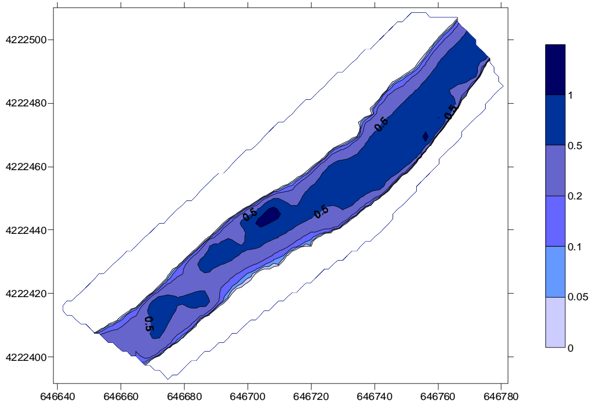
Figura 11. Calados para el caudal 2,2 m 3 /sg en tramo representativo de la masa de agua ES0701010113
