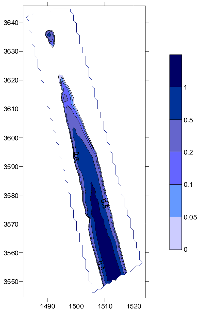
Figura 17. Calados para el caudal de los modelados donde se observa pérdida de continuidad en tramo de la masa de agua ES0701010301 ( 0,1 \text{ m}^3/\text{sg} )
