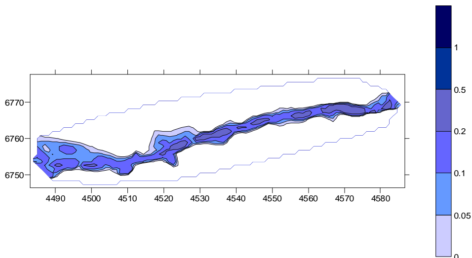
Figura 25. Calados para el caudal menor de los modelados 0,25 m 3 /sg en tramo de la masa de agua ES0701011103, donde no se observa pérdida de continuidad
