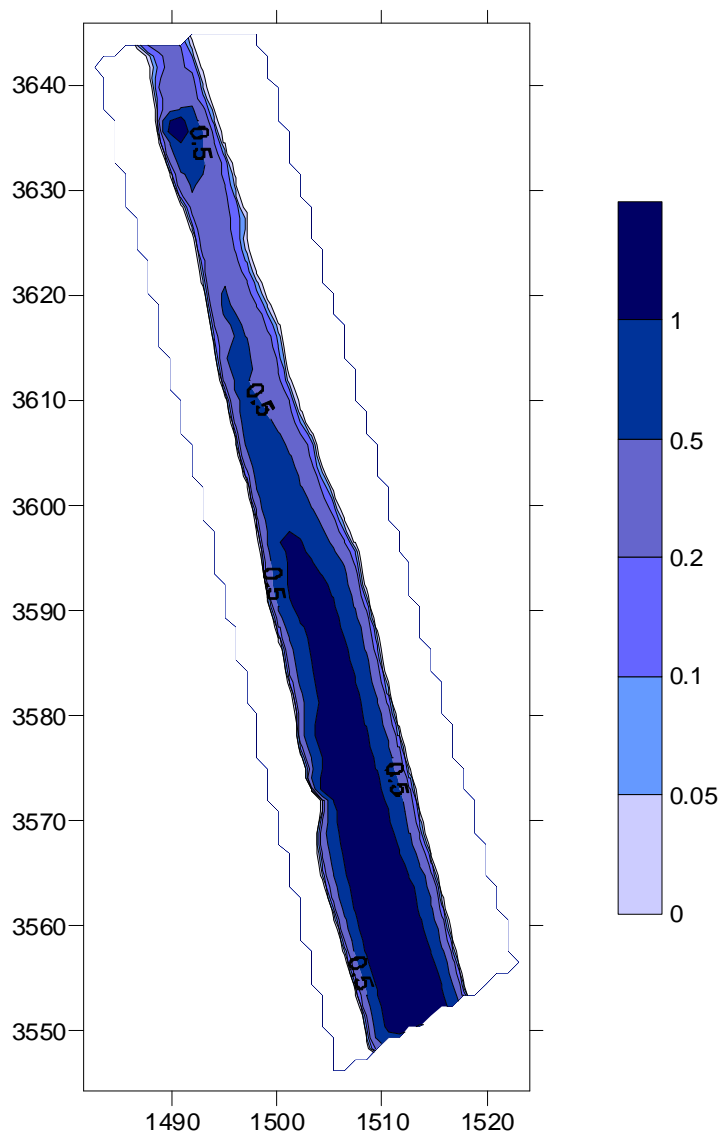
Figura 16. Calados para el caudal 0,15 m 3 /sg en tramo de la masa de agua ES0701010301
