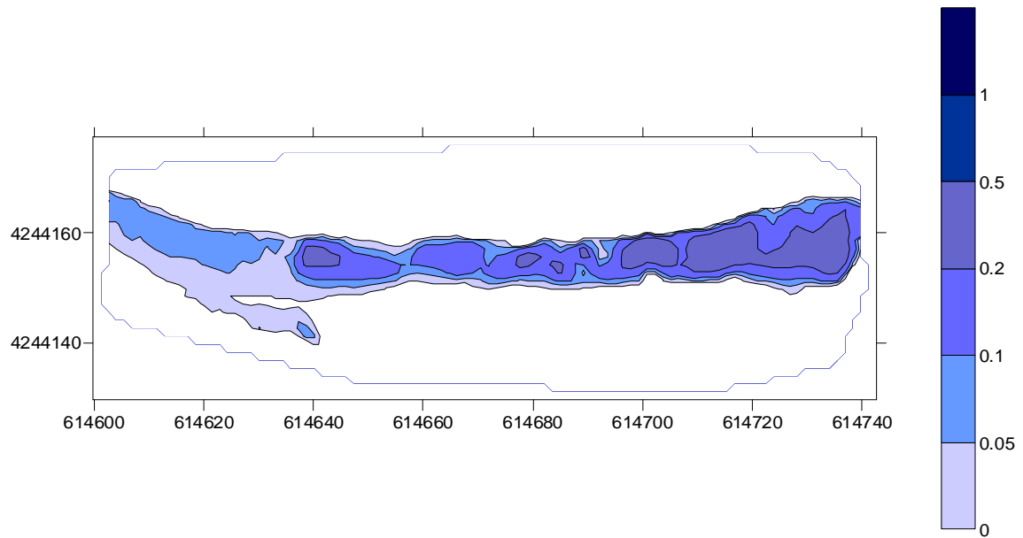
Figura 7. Calados para el caudal de los modelados anterior al que presenta la pérdida de continuidad en tramo de la masa de agua ES0701010109 ( 0,2 \text{ m}^3/\text{sg} )
