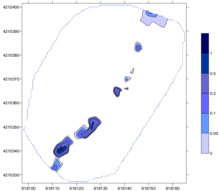
Figura 36. Calados para el caudal 0,1 m 3 /sg, que coincide con el caudal de los modelados en el que se observa pérdida de continuidad, en el tramo de la masa de agua ES0701012304
