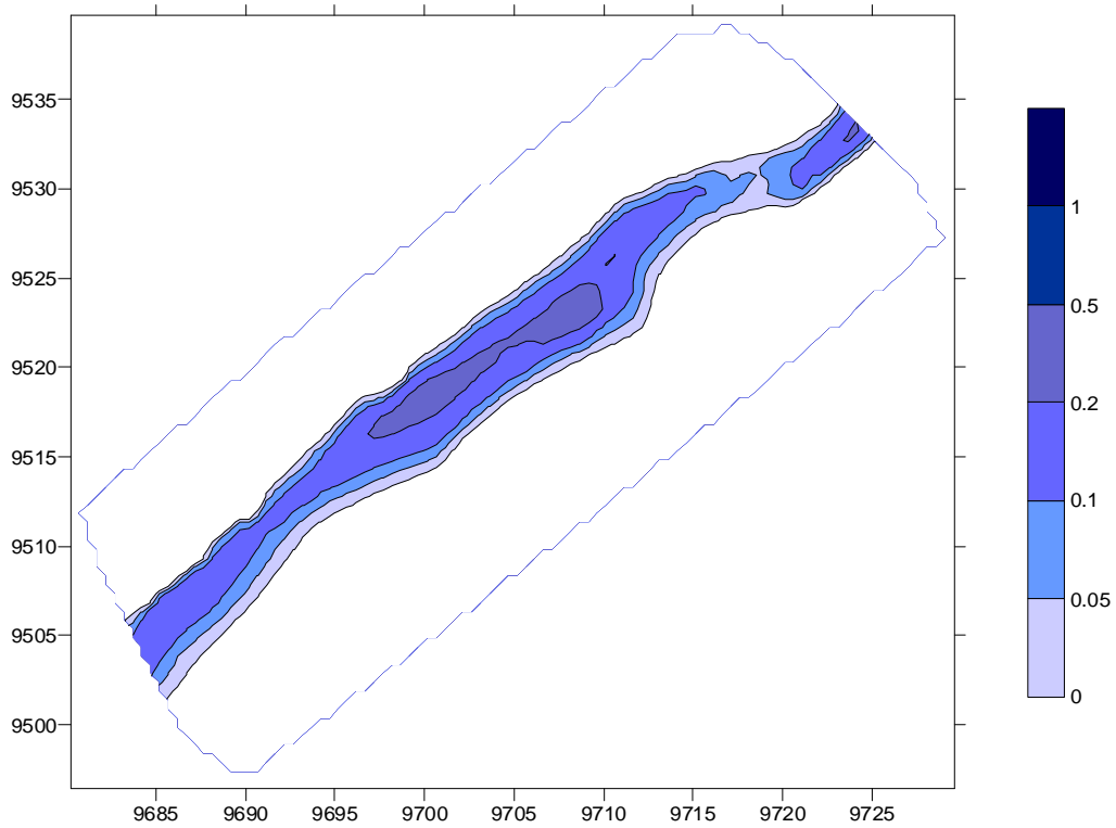
Figura 33. Calados para el caudal 0,11 m 3 /sg en tramo de la masa de agua ES0701012002
