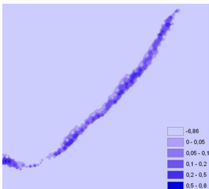
Figura 15. Calados para el caudal de los modelados donde se observa la pérdida de continuidad en tramo de la masa de agua ES0701010203 (0,01 m 3 /sg)
