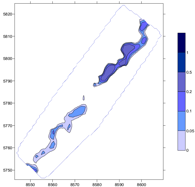
Figura 3. Calados para el caudal de los modelados que produce la pérdida de continuidad en el tramo de la masa de agua ES0701010101 ( 0,05 \text{ m}^3/\text{s} )
