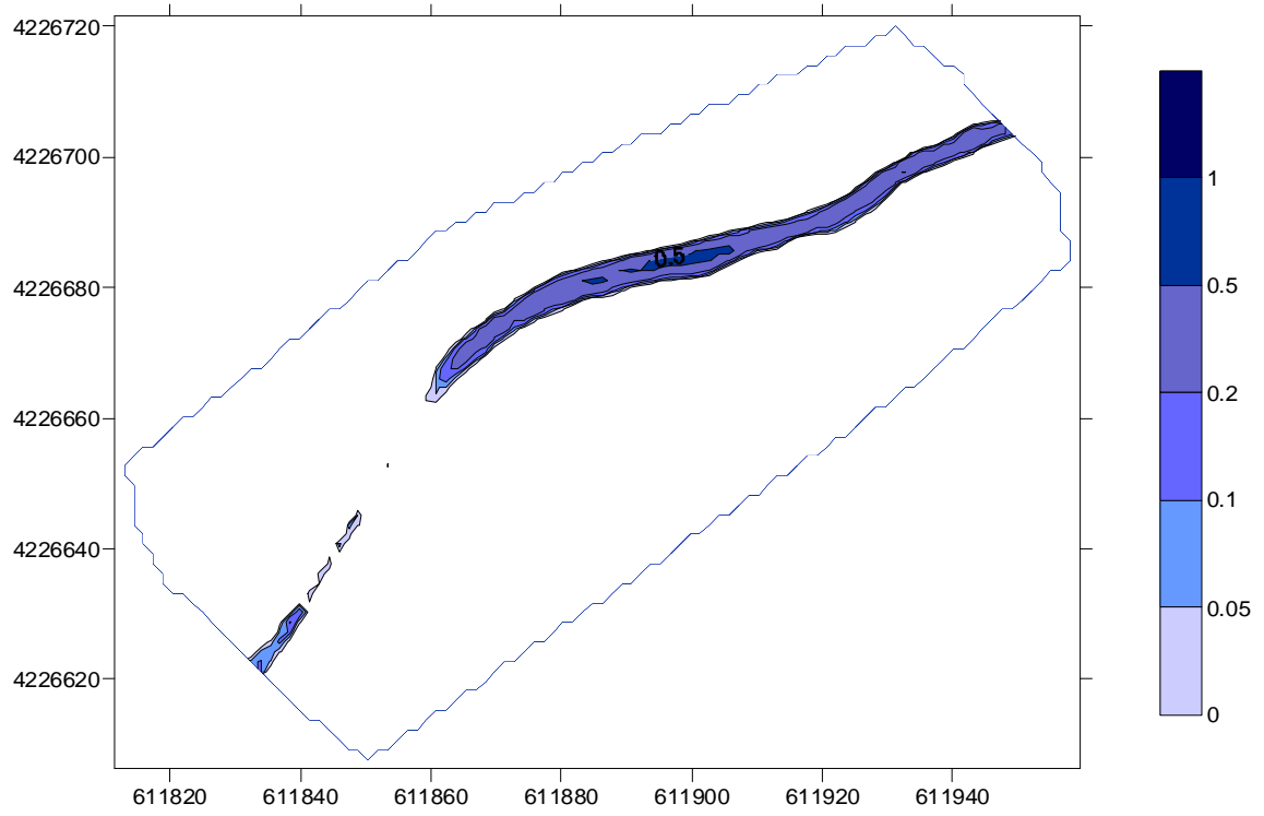
Figura 32. Calados para el caudal de los modelados donde se observa pérdida de continuidad en tramo de la masa de agua ES0701011903 ( 0,05 \text{ m}^3/\text{sg} )
