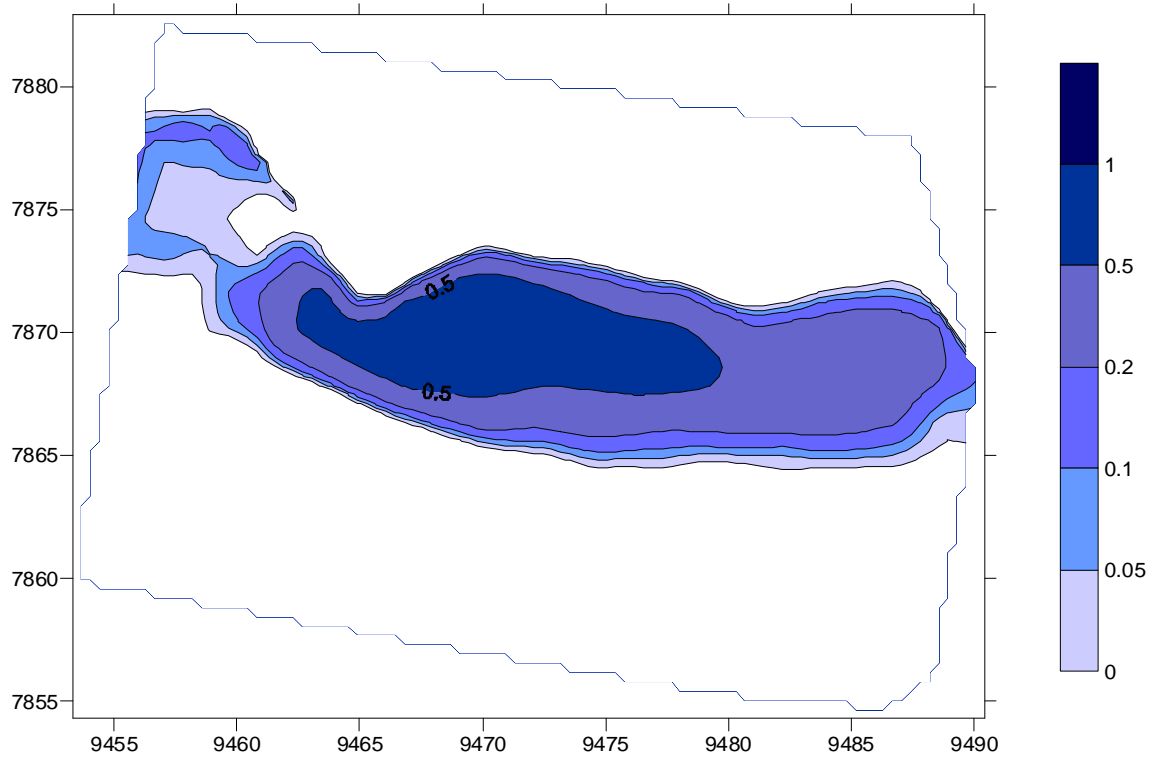
Figura 22. Calados para el caudal de los modelados anterior al que presenta pérdida de continuidad en tramo de la masa de agua ES0701010401 ( 0,1 \text{ m}^3/\text{sg} )
