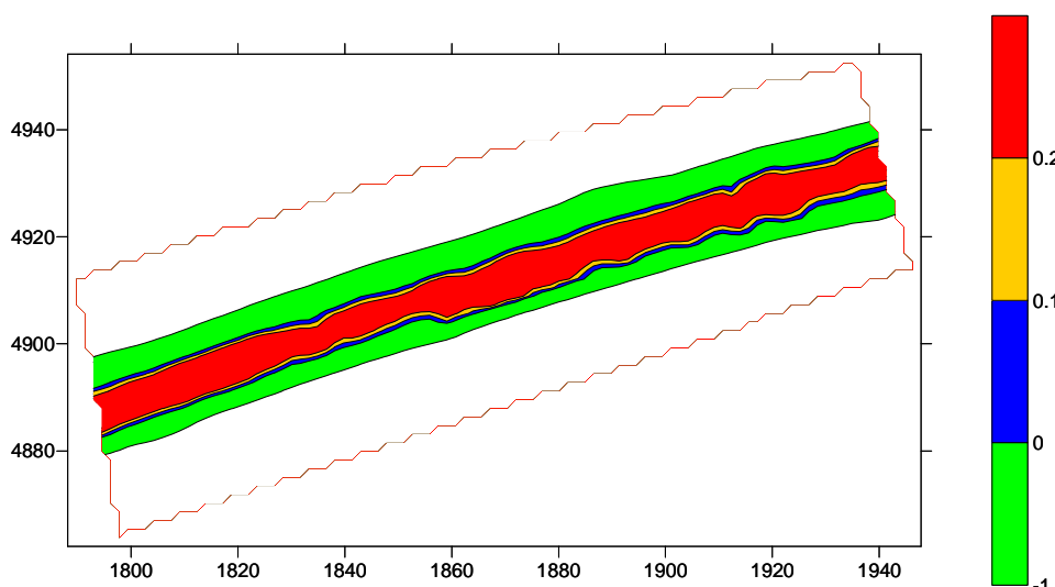
Figura 39. Calados para el caudal 1 m 3 /sg en tramo de la masa de agua ES0702080115
