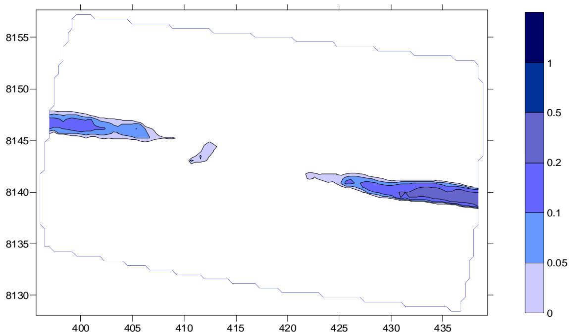
Figura 28. Calados para el caudal de los modelados donde se observa pérdida de continuidad en tramo de la masa de agua ES0701011801 y ES0701011802 ( 0,05 \text{ m}^3/\text{sg} )
