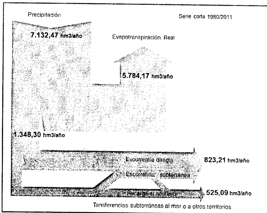
Figura 6. Los mismos componentes del ciclo hídrico en el Segura de la figura anterior calculados en volumen (hm³/año).
